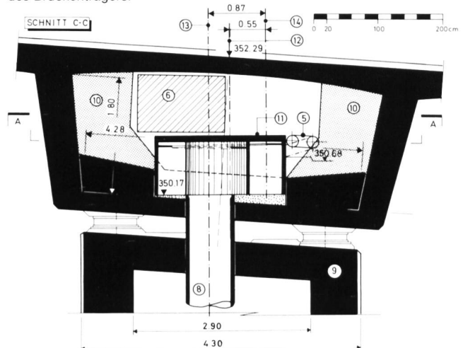
Bild 4. Querschnitt C-C.
