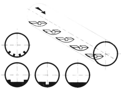
Bild 4. Fischdurchlass. Rohrströmung mit freiem Spiegel, durch Querswellen verlangsamt.
