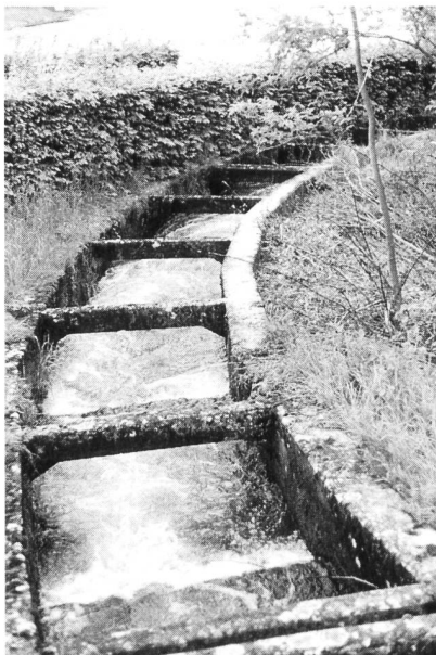
Bild 11. Beckenpass beim Aarekraftwerk Hagneck.
