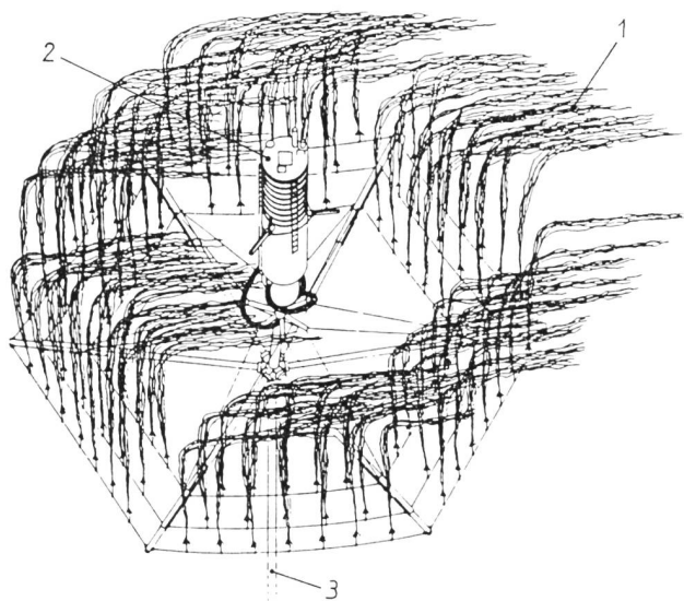
Bild 1. Die Kelpversuchsfarm vor Laguna Beach (Kalifornien). 1 Riesenkelp (Macrocystis); 2 Boje mit Instrumenten, Motoren, Pumpe; 3 Nährstoffleitung, 450 m lang, Durchsatz 30000 l/min. Der Aussendurchmesser der Struktur beträgt etwa 32 m (aus: W. J. North, V. A. Gerard, J. S. Kuwabara, W. M. Keck, Caltech: «Biomass Production by Freshwater Marine Macrophytes», 1980).
