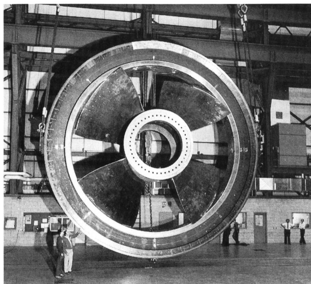
Bild 2. Das Laufrad der Strafloturbine des Gezeitenkraftwerks Annapolis Royal. Laufrad mit 7,6 m Durchmesser und 4 festen Schaufeln (Propellerturbine). Gefälle: 1,4 bis 7,1 m; Nennfallhöhe 5,5 m; 378 m 3 Wasser pro Sekunde; 50 U/min; Nennleistung: 17,8 MW. Der fest auf den Schaufeln angebrachte Generator-Rotorring ist deutlich ersichtlich (Foto: Sulzer-Escher Wyss, Zürich).
