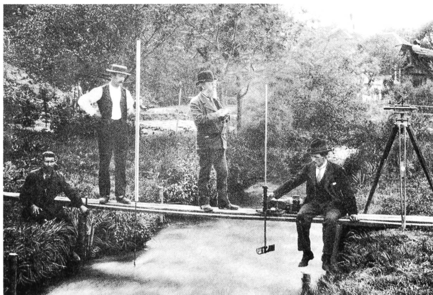
Bild 1. Abflussmessung einst...
