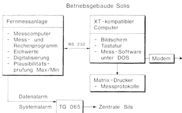
Bild 4. Der Fernmessanlagenteil im Betriebsgebäude Solis.
