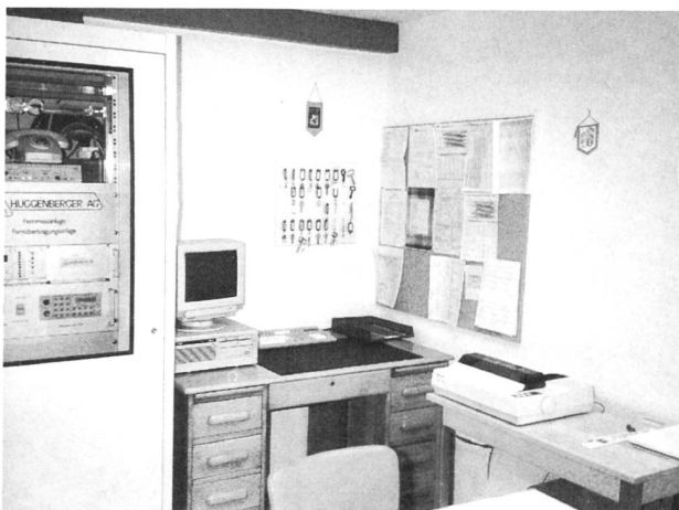
Bild 5. Der Fernmessanlagenteil im Betriebsgebäude Solis. Links im Schaltschrank der Messcomputer der Firma Huggenberger AG und darüber das PTT-Modem für die Verbindung nach Zürich. Auf dem Schreibtisch der XT-kompatible PC mit Bildschirm, Tastatur und daneben der Matrix-Drucker.
