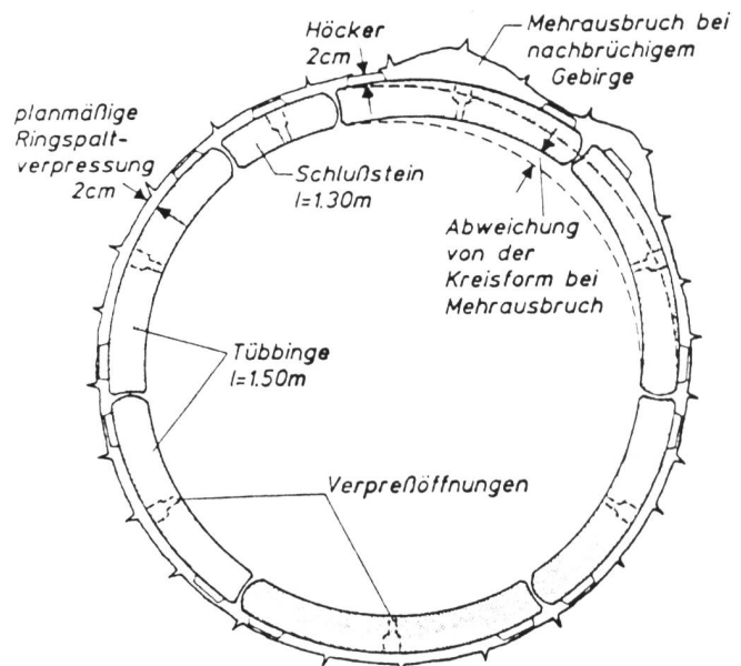
Bild 4. Spreitzübbing (flexible expanded lining).
