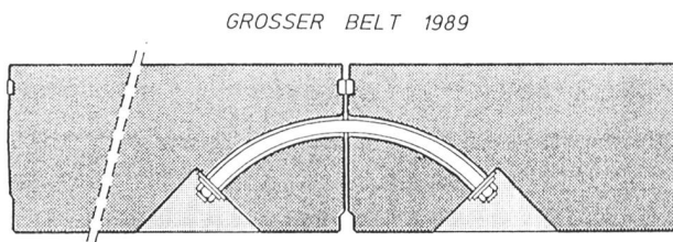
Bild 3. Ringfugen mit Längsverraubung bei Stahlbetontübbing.
