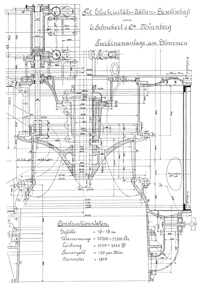
Bild 3. Glommen-Zylinderschütze, erstmals Ausbildung einer besonderen Fussform der Schütze zur Verminderung strömungserregter Schwingungen, P = 3850 HP, H = 18 m, aus [2].
