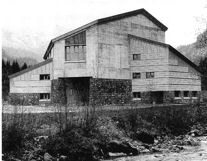
Bild 1. Standfestigkeit gegenüber drohenden Naturgewalten lässt die Form des neuen Kraftwerksgebäudes Kandergrund der BKW sichtbar werden (Eingangspartie von Nordwesten).
