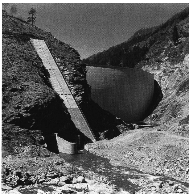
Figure 2. La retenue de Malvaglia à sec lors de la construction. De gauche à droite: la vidange de fond, la prise d'eau, le barrage-voûte.
