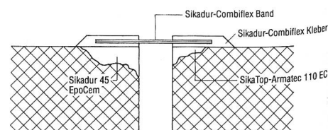
Bild 6. Sanierung von undichten und beschädigten Fugen.
