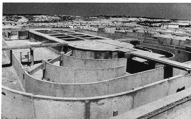
Bild 7. Bau einer Kläranlage in Rishon, Israel. Fugenabdichtungen: Sikaflex T 68 NS.
