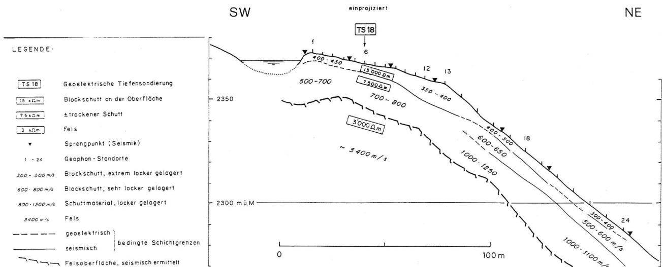
Bild 2. Geophysikalische Eigenschaften des Moränendamms am Sidelengletscher (Gerental/Obergoms). Die Sondierungen wurden 1988 im Rahmen der «Ursachenanalysen Hochwasser 1987» durchgeführt.
