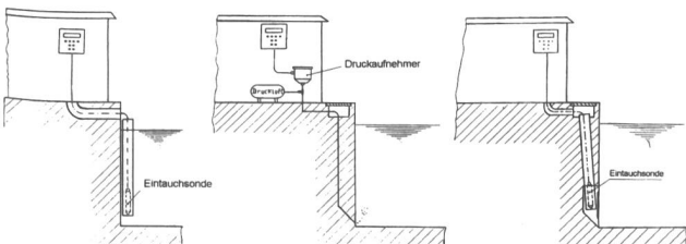
Bild 4, links. Messwertaufnahme (Eintauchsonde) am Messort, aufputz.
