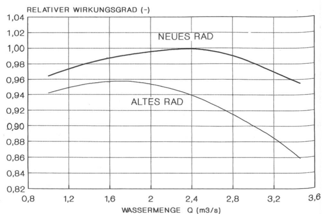
Bild 4. Vergleichsmessung altes/neues Laufrad der Anlage Küblis bei einer Nettofallhöhe von 365 m.
