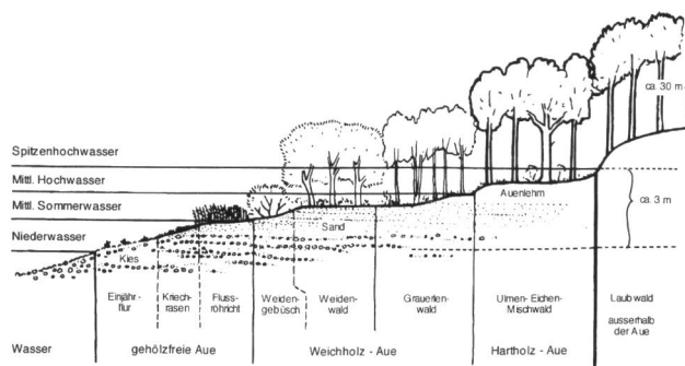
Bild 1. Schematischer Querschnitt durch eine Aue (aus Ellenberg 1982).
