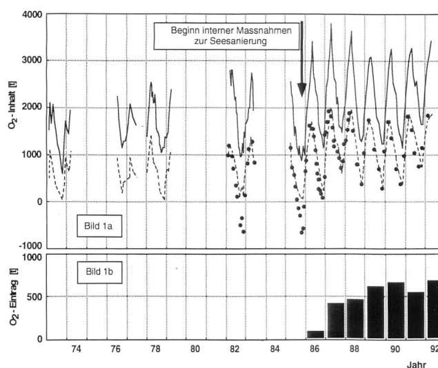
Bild 1. a) Sauerstoffinhalt des Hallwilersees in Tonnen im gesamten See (ausgezogene Linie) und im Tiefenwasser unterhalb 13 m Tiefe (durchbrochene Linie). Die Punkte bezeichnen den «theoretischen» Sauerstoffinhalt im Tiefenwasser nach Abzug des Sauerstoffbedarfs zur Oxidation von gelösten, reduzierten Substanzen. b) Die während des Sommers ins Tiefenwasser eingetragenen Sauerstoffmengen.
