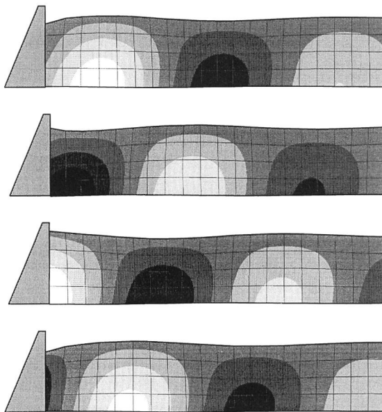
b) Kompressibles Wasser, harmonische Mauerbewegung, f_{mv}/f_s = 1.5
