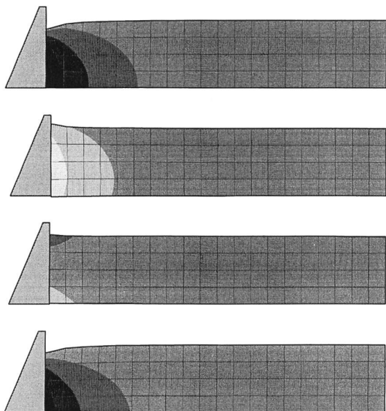
a) Kompressibles Wasser, harmonische Mauerbewegung, f_{mv}/f_s = 0.8
