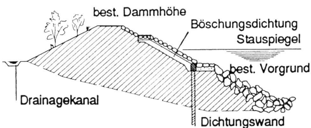
Bild 3. Dammquerschnitt (modifizierte Figur B 11, S. 30, Hauptbericht).
