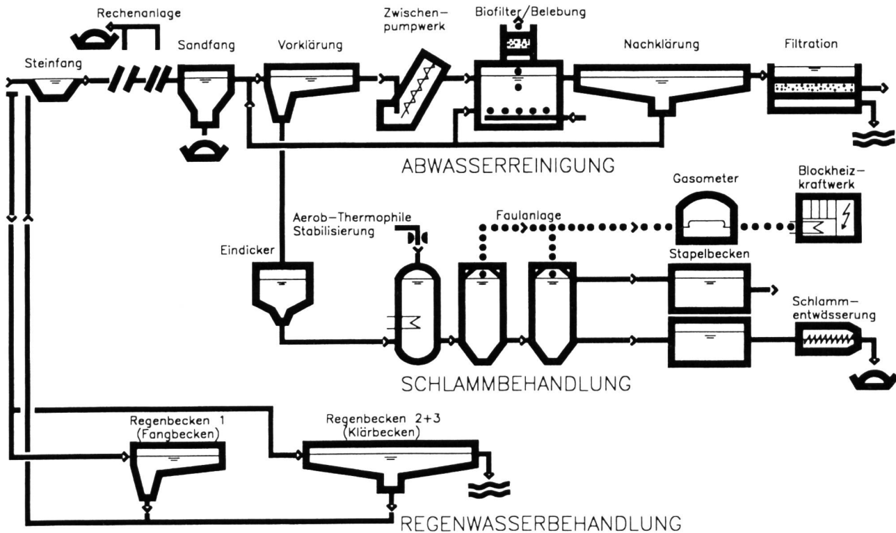
Bild 3. Funktionsschema der ARA Ergolz 1.
