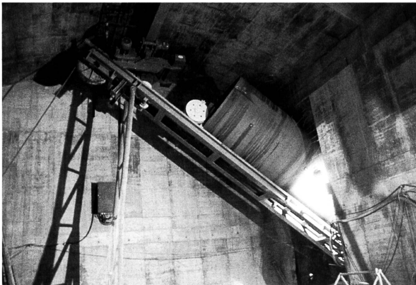
Bild 4. Kippvorrichtung in der Schieberkammer für die Montage der Panzerrohre im schrägen Teil des Druckschachtes.
