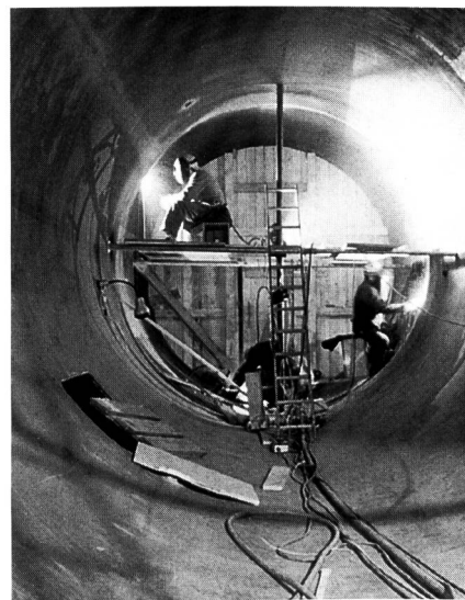
Bild 6. Schweissarbeiten an der Panzerung beim Druckschachtfuss.
