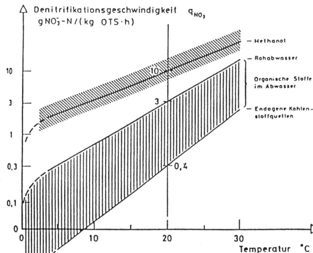
Bild 1. Denitrifikationsgeschwindigkeit als Nitratabnahme (g Nitrat-Stickstoff pro kg organische Trockensubstanz und Stunde, g\ NO_3-N/(kg\ OTS \cdot h) ) in Abhängigkeit von Temperatur und Kohlenstoffquelle. Bei natürlichen Kohlenstoffquellen (vertikal gestrichelt) nimmt die Denitrifikationsgeschwindigkeit mit abnehmender Temperatur stark ab. Bei schlecht verfügbaren Kohlenstoffquellen (untere Gerade der gestrichelten Fläche) wird die Denitrifikationsleistung gering.
