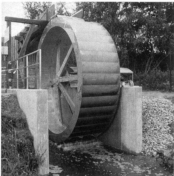
Turas-Wasserrad mit 4,80 m Durchmesser im Ablauf des Klärwerks Warendorf.
