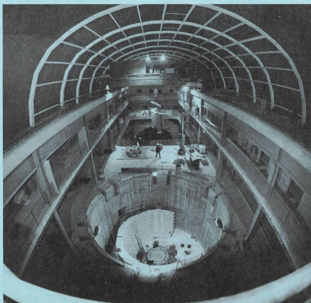
Pose d'une carcasse statorique sur le groupe 3 de l'usine de Bieudron (Photo H. Preisig , 10 janvier 1997) Statormontage Gruppe 3 in der Kavernenzentrale Bieudron (Foto H. Preisig , 10. Januar 1997)
