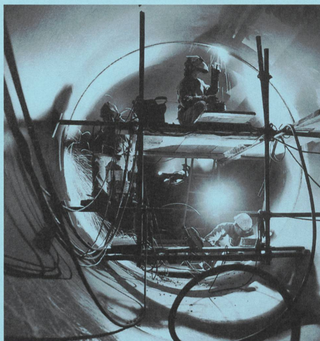
Schweissen im Druckschacht, Abzweigung zur Gruppe 1 in der Kavernenzentrale Bieudron (Foto H. Preisig, 11. März 1997) Soudure de la bifurcation de la conduite forcée reliant le groupe 1 de la centrale souterraine de Bieudron (Photo H. Preisig, 11 mars 1997)
