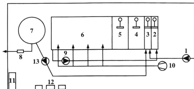
Bild 1. Pilotanlage. 1 Zulaufpumpe, 2 Gelöstsauerstoff Abbauzone, 3 Mischzone, 4 Denitrifikationszone 1, 5 Denitrifikationszone 2, 6 Nitrifikationszone, 7 Nachklärung, 8 Durchflussmesser, 9 interne Rezirkulation, 10 Gebläse, 11 Steuer- und Regelschranke, 12 Instrumente, 13 Rücklaufschlammpumpe.
