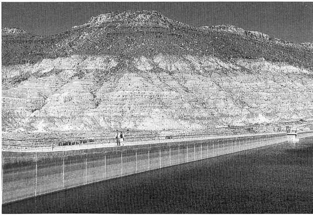
Bild 4. Ansicht des Quail Creek South Dam: a), links, Wasserseite aus mittels Gleitschalungsfertiger eingebautem konventionellem Beton mit Entnahmeturm (rechts); b), rechts, Luftseite aus ungeschaltem Walzbeton mit niedriger ausgebildeter Mauerkrone aus konventionellem Beton im Bereich der Not-HWE und RCC-Sohlbefestigung am Mauerfuss.
