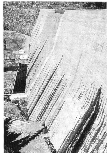
Bild 2, links. Nichtgeschalter Walzbeton auf der Luftseite des Quail Creek South Dam in Utah, mit einem mittleren Bindemittelgehalt von 133 \text{ kg/m}^3 und einer Schichtdicke von 30 cm.
