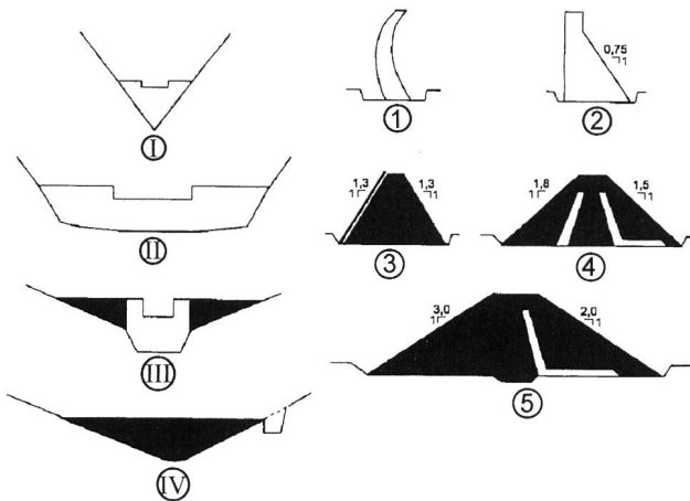
Bild 6. a) Talformen: (I) Kerbtal, (II) Trogtal, (III) Canyon plus Muldentale, (IV) Muldentale; b) Talsperrentypen: ① Doppelt gekrümmte Bogenmauer (Kuppelmauer), ② Gewichtsstauwehr, ③ Steinschütt-damm mit Betonoberflächendichtung, ④ Steinschütt-Zonendamm, ⑤ Erdschütt-damm mit Oberflächen- oder Innendichtung.
