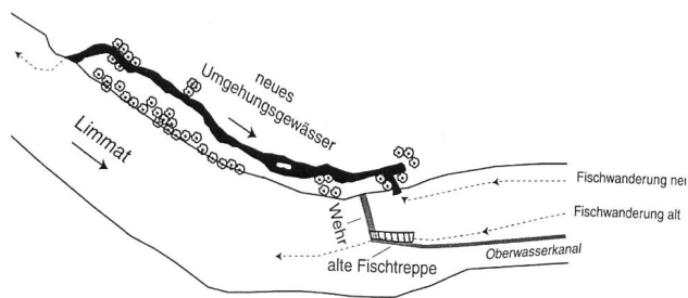
Bild 3. Situationsskizze.
