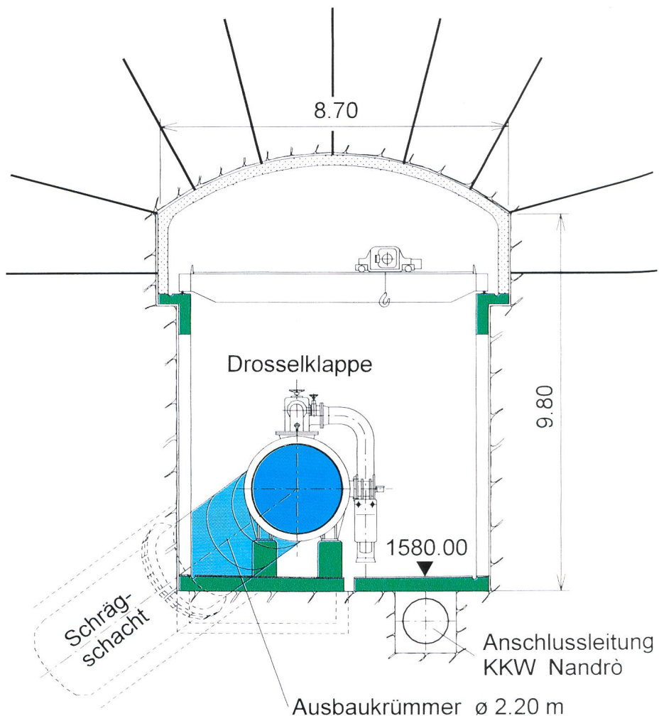
Bild 7. Querschnitt Kaverne.
