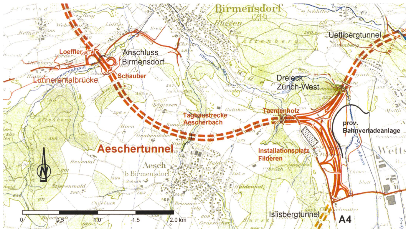
Bild 1. Situation Aeschertunnel.
