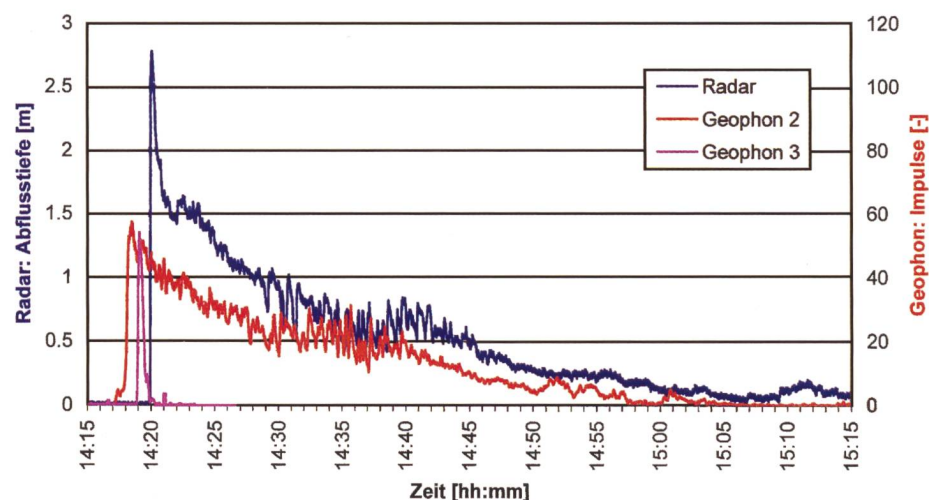
Bild 9. Murgang im Illgraben vom 28. Juni 2000: Zeitlicher Verlauf der Abflusstiefe aus den Radarmessungen im Vergleich zu den Aufzeichnungen der Erschütterungsintensität durch zwei Geophonsensoren.
