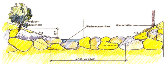
Bild 8. Querprofil der Sohlswelle.
