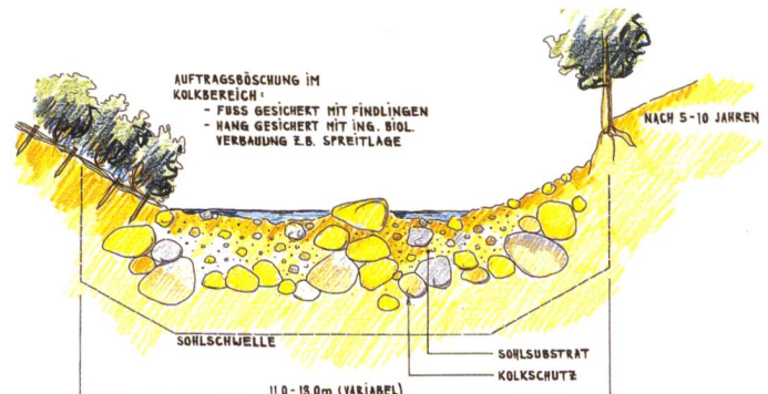
Bild 9. Querprofil zwischen den Sohlswellen.
