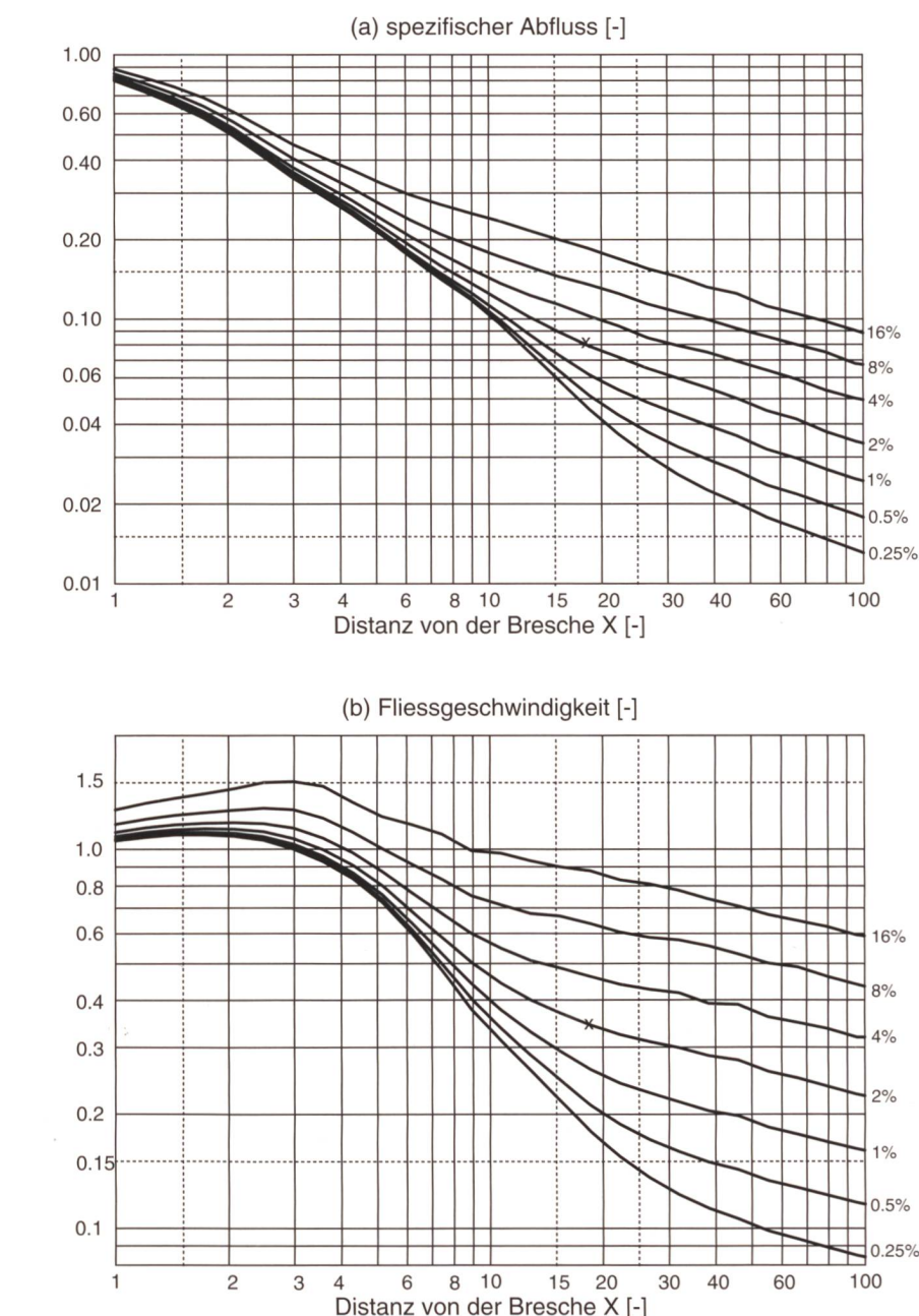
Diagramm A. Längenprofil entlang der Strahlachse für spezifischen Abfluss (a) und Fliessgeschwindigkeit (b).
