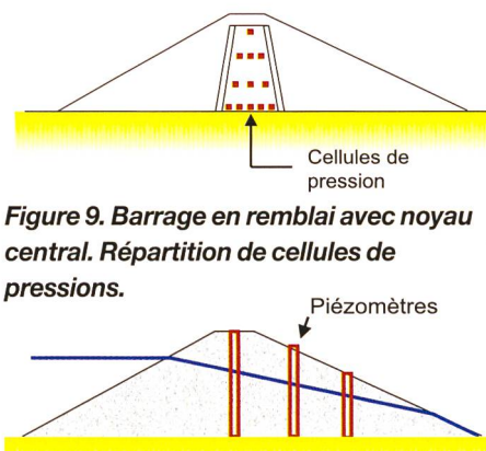
Figure 9. Barrage en remblai avec noyau central. Répartition de cellules de pressions.
