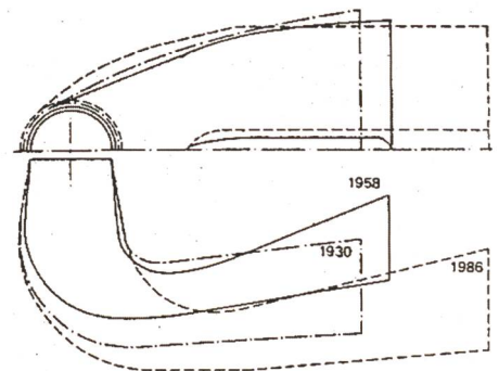
Bild 2. Historische Entwicklung der Saugrohrformen von Francisturbinen (aus [1]).
