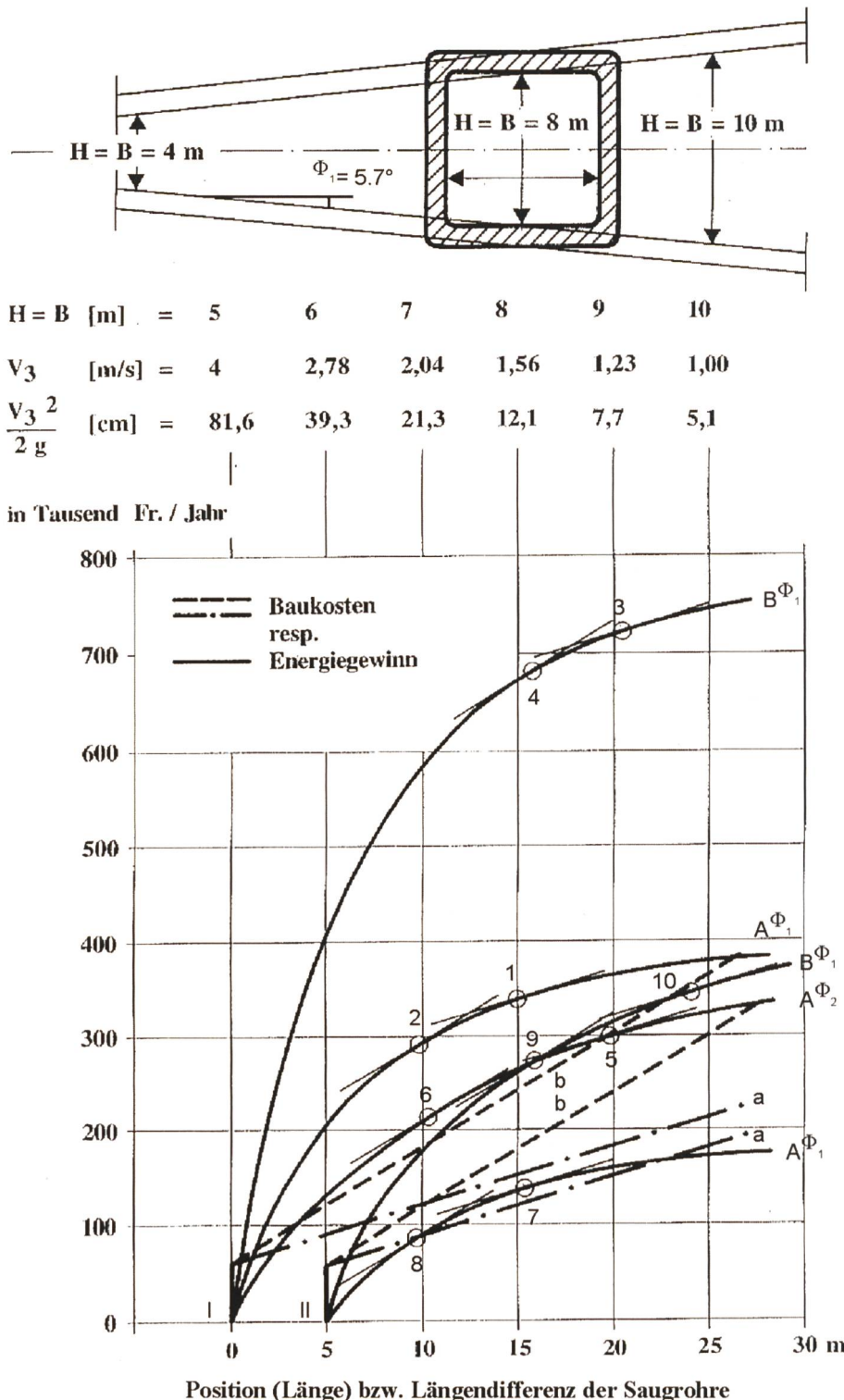
Bild 4. Energiegewinn und Baukosten für verschiedene Saugrohrverlängerungen.
