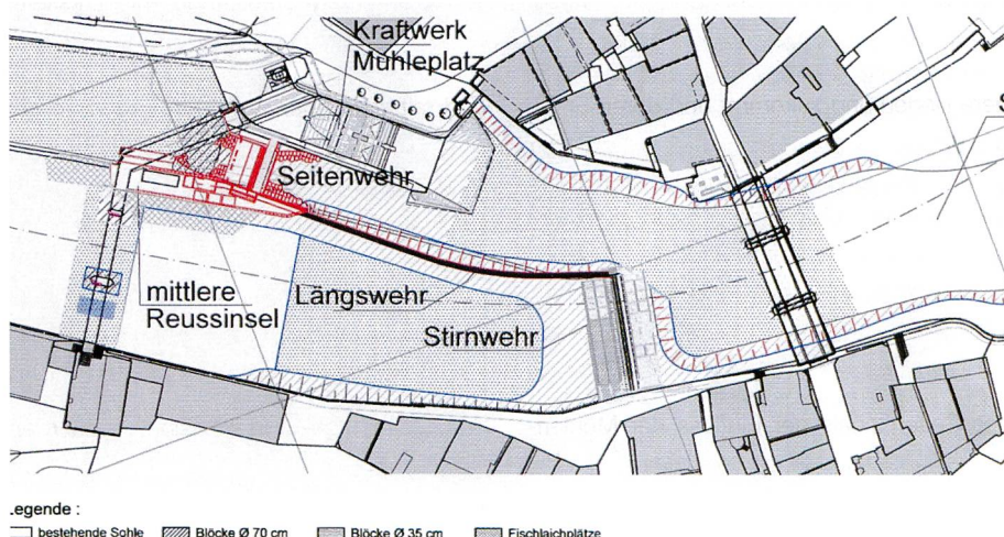
Bild 14. Gesamtsituation der Reusswehranlage mit eingetragenen Bauwerken, der Sohlenabsenkung und der Sohlensicherung mit Blockteppich.
