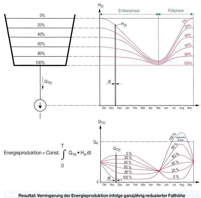
Bild 10. Bruttogefälle H(t) und mittlerer Tages-Turbinenvolumenstrom Q_{T(t)} in Abhängigkeit des prozentualen Freihaltevolumens.
