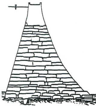
Bild 5. Die Lower-Crystal-Springs-Gewichtsmauer in unmittelbarer Nähe der San-Andreas-Verföhrung hat die starken Erschütterungen des San-Francisco-Erdbebens von 1906 schadlos überstanden. Die 44,5 m hohe Mauer besteht aus verzahnten Betonblöcken, und bei starker seismischer Beanspruchung können sich kurzfristig einige der Fugen öföfen. Als 1887 mit dem Bau dieser Mauer begonnen wurde, war dies weltweit die grösste Staumauer. Die Mauer wurde 1911 erhöht (Foto: City of San Francisco).
