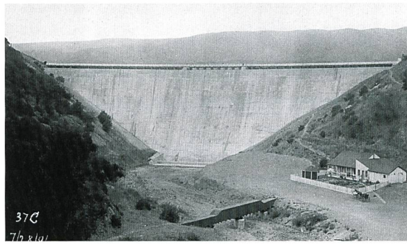
Bild 5. Die Lower-Crystal-Springs-Gewichtsmauer in unmittelbarer Nähe der San-Andreas-Verföhrung hat die starken Erschütterungen des San-Francisco-Erdbebens von 1906 schadlos überstanden. Die 44,5 m hohe Mauer besteht aus verzahnten Betonblöcken, und bei starker seismischer Beanspruchung können sich kurzfristig einige der Fugen öföfen. Als 1887 mit dem Bau dieser Mauer begonnen wurde, war dies weltweit die grösste Staumauer. Die Mauer wurde 1911 erhöht (Foto: City of San Francisco).
