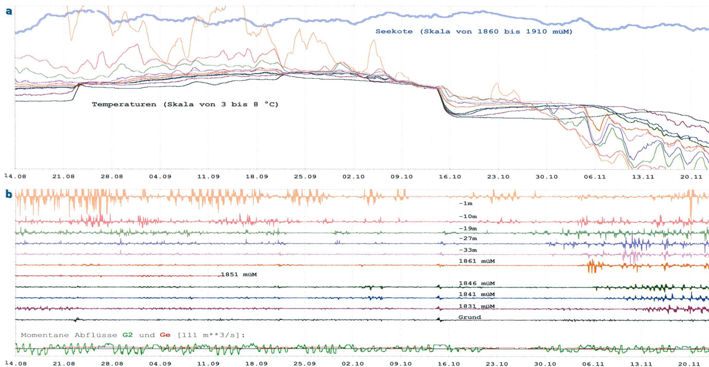
Bild 8. Temperaturdaten im Grimselsee vor der Spittellamm Sperre und momentane KWO-Abflüsse von Montag, 14. August, bis Mittwoch, 22. November 2000.
