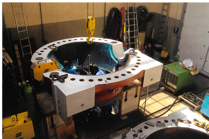
Bild 9. Verschweissen des Ersatzringes.
