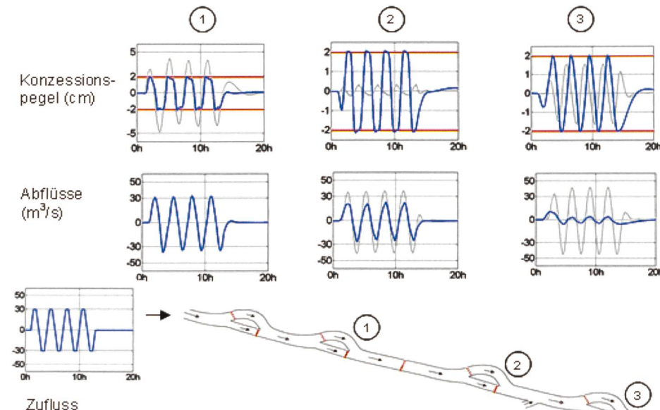
Bild 8b. Pegel und Durchflüsse bei einer sinusförmigen Zuflussschwankung (hell: lokale PI-Regler, dunkel: MPC).
