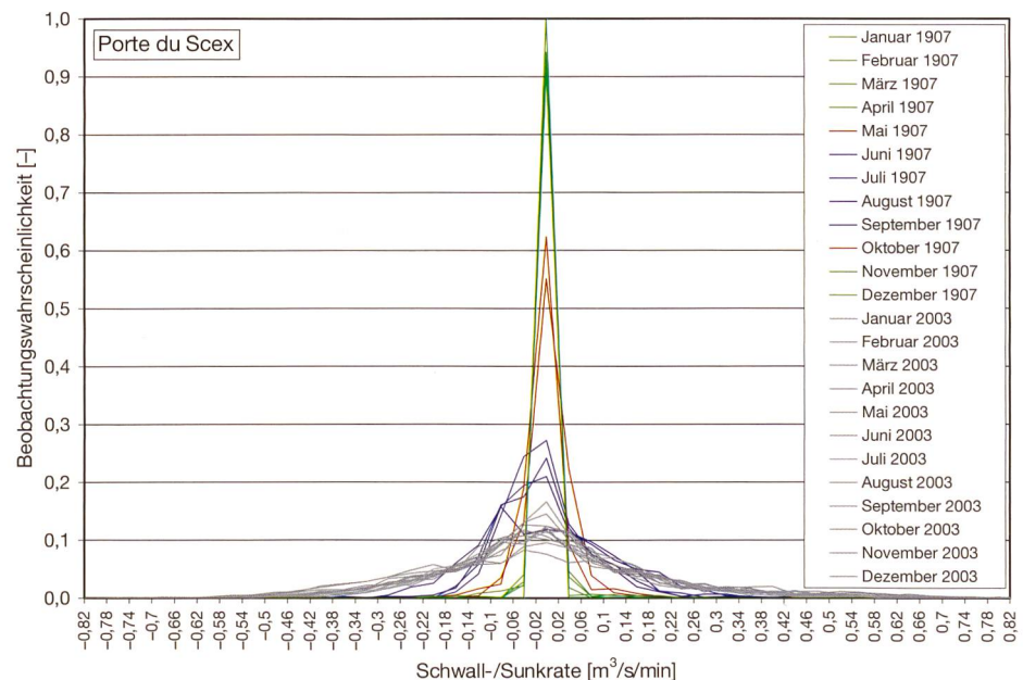
Bild 14. Monatliche Beobachtungswahrscheinlichkeiten der Schwall- und Sunkraten in der Station Porte du Scex für 1907 und 2003. Grün: Wintermonate 1907 (November–April). Rot: Übergangsmonate 1907 (Oktober, Mai). Blau: Sommermonate 1907 (Juni–September). Grau: Alle Monate 2003.
