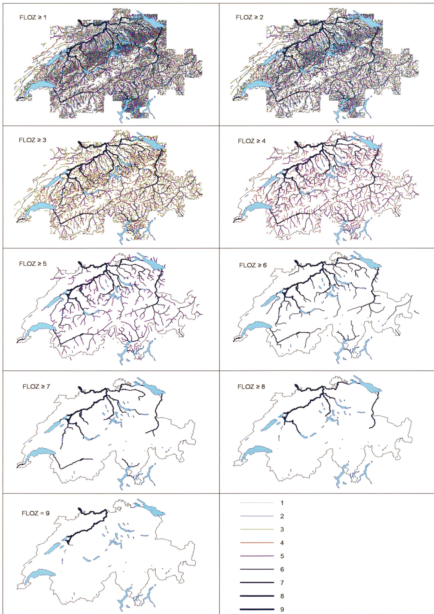
Bild 2. Nach Flussordnungszahl (FLOZ) aufgliedertes Gewässernetz der Schweiz.
