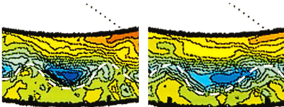
Bild 9. Strömungsverhältnisse mit der Geometrie der optimierten Ausbuchtungen des Blockwurfes mit variabler Neigung ( Q = 100 \text{ l/s} , Lage zwischen 48^\circ und 60^\circ in Kurve).
