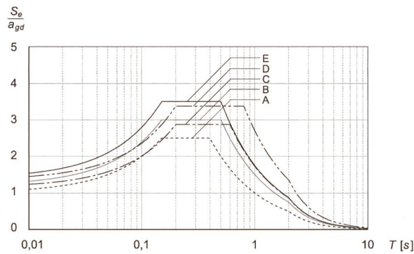
Bild 2. Elastische Beschleunigungsantwortspektren der SIA-Norm 261 (2003) für 5%-Dämpfung für verschiedene Baugrundklassen (A = Fels) und einer Spitzenbodenbeschleunigung von a_{gd} (Wiederkehrperiode: 475 Jahre).
