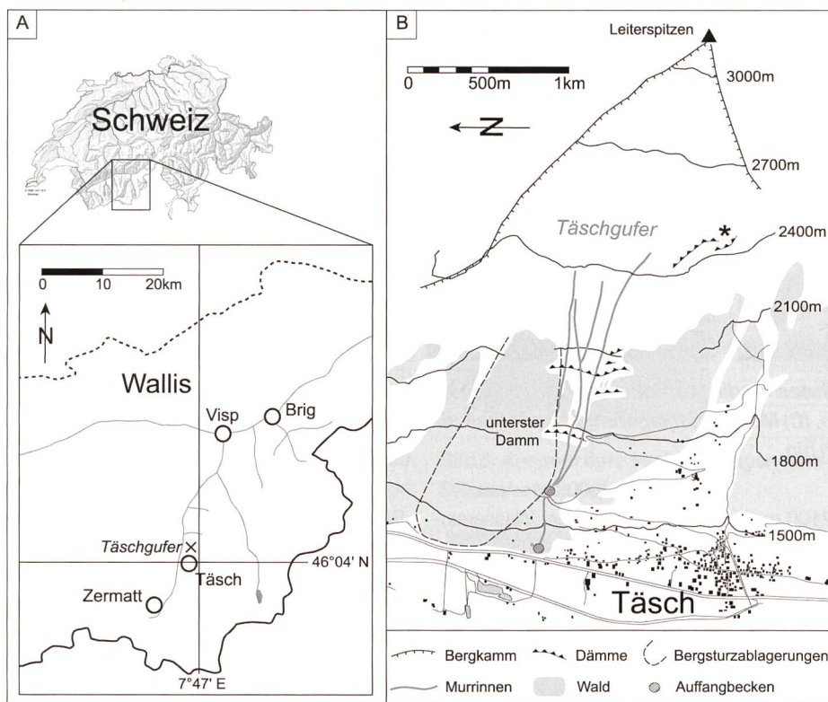
Bild 1. Das Untersuchungsgebiet Täschgufer befindet sich im südlichen Murtal. Der Hang weist mehrere aktive Murrinnen und zahlreiche Schutzdämme gegen Steinschlag auf, wobei sich der unterste Damm bei 1780 m ü.M. befindet. Beim Bau der obersten Dämme wurde Permafrost gefunden (*).
