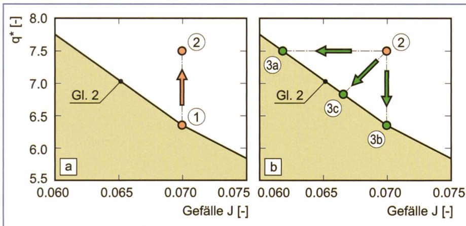
Bild 6. Konzept der Anpassung der Gerinnesohle, wenn der spezifische Abfluss einen Grenzwert der Stabilität überschreitet. Die durchgezogene Linie entspricht hier Gleichung (2) nach Aberle (2000).
