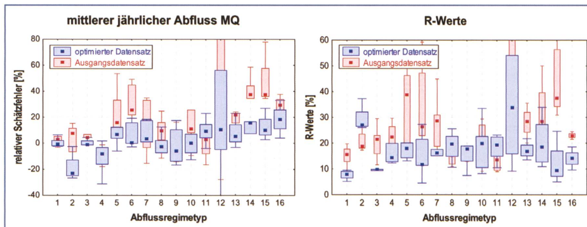
Bild 6. Nach Abflussregimtypen differenzierte Analyse der Schätzgenauigkeit; die Box-plots geben auf der Basis der Validationsstationen pro Abflussregimtyp die Verteilung (Median, 25/75% Quantil und Min/Max) der Schätzfehler wider.
