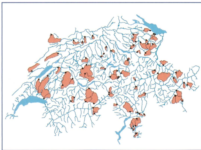
Bild 3. links: Karte mit der räumlichen Lage der Validationsstationen und ihren Einzugsgebieten (ohne diejenigen des Abflussregimetyps 12); rechts: Verteilung der Validationsstationen auf die 16 Abflussregimetypen.
