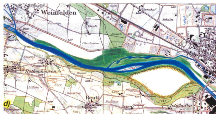
Bild 3. Beispiel von Wasserbauvarianten für das Fallbeispiel Weinfelden-Bürglen. Die Kantonsvariante (a) beinhaltet ein Rückhaltebecken für den Hochwasserschutz und eine Aufweitung des Flussbetts, die Variante Naturreservat (b) setzt auf ökologische Aufwertung, die Minimalvariante (c) beinhaltet eine Verdoppelung des Flussbetts, und die Kombinationsvariante (d) verbindet die Ziele «Hochwasserschutz», «Erhaltung Landwirtschaftsland» und «ökologische Aufwertung». Quelle: Hostmann (2005).
