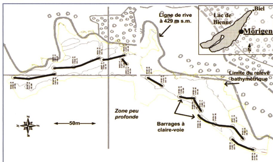
Figure 1. Le site de Mörigen sur le lac de Biene avec ses mesures de protection.
