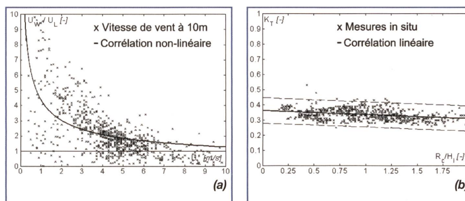
Figure 2. Mesures réalisées in situ: (a) vitesses de vents à Neuchâtel ( U_L ) comparées à celles mesurées à Mörigen ( U_w ); (b) coefficient de transmission K_T des barrages à claire-voie à Mörigen sur le lac de Biene en fonction de la revanche relative R_c/H_1 (BFH 2005).
