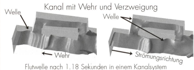
Flutwelle nach 1.18 Sekunden in einem Kanalsystem
