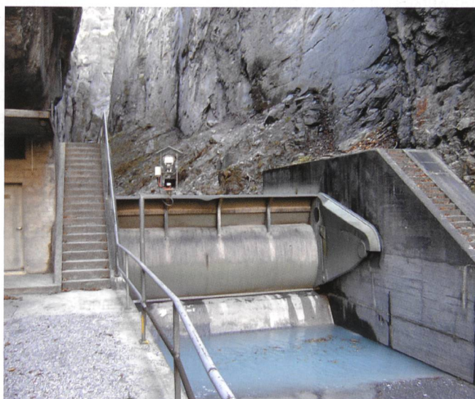
Bild 8. Falls der Muttsee aufgestaut wird, so wird als Ausgleichsmassnahme dazu die Fassung Linth Schlucht aufgegeben und rückgebaut.
